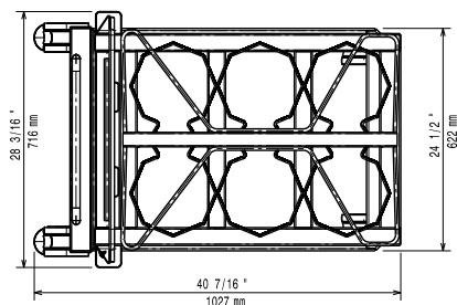
Boven aanzicht
